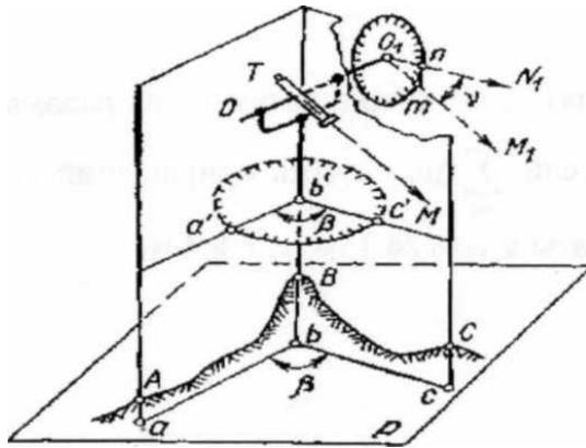
Рис. VI.1. Принцип измерения горизонтальных и вертикальных углов.
